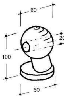
Art. 35-00002 Sfera con foro Ø60 Raw ball Ø60 with eyelet (Kg.1,243)
