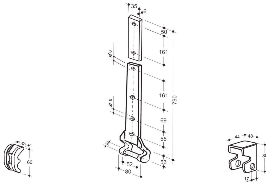
Art. 31-00042 (Kg.0,100) Paletta per cerniera Raw locking plate
