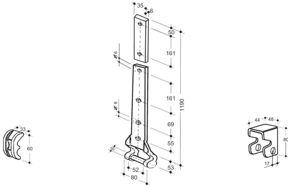
Art. 31-00042 (Kg.0,100) Paletta per cerniera Raw locking plate
